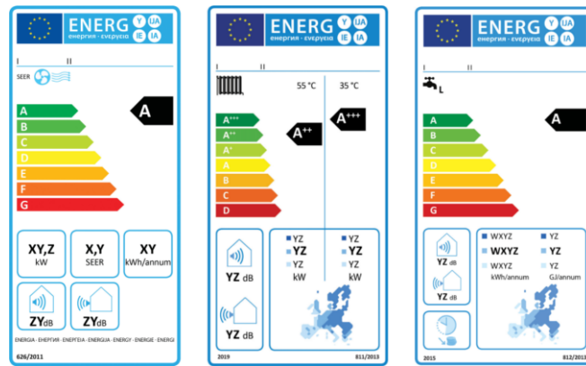
Abbildung 1: Muster des Energielabels für Klimageräte (Verordnung (EU) Nr. 626/2011), für Raumheizungen mit Wärmepumpe (Verordnung (EU) Nr. 811/2013) und für Warmwasserbereiter mit Wärmepumpe (Verordnung (EU) Nr. 812/2013). Der Schallleistungspegel (außen) wird symbolisiert dargestellt ( ) und als „ZY dB“ bzw. „YZ dB“ angegeben.
